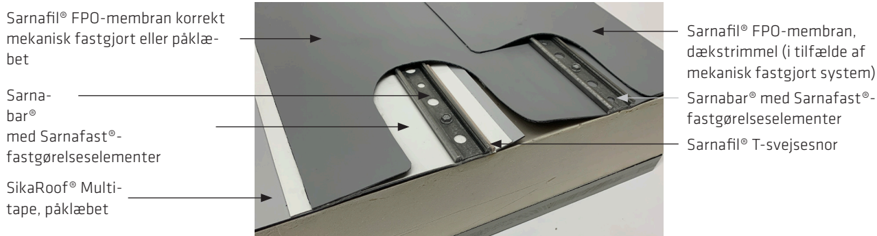
4. Automatisk varmluftsvejsning af Sarnafil® FPO-membran på SikaRoof® Multitape.
